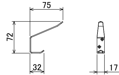
ステンレス帽子掛(S=1/5) SUS-304-ヘアライン
